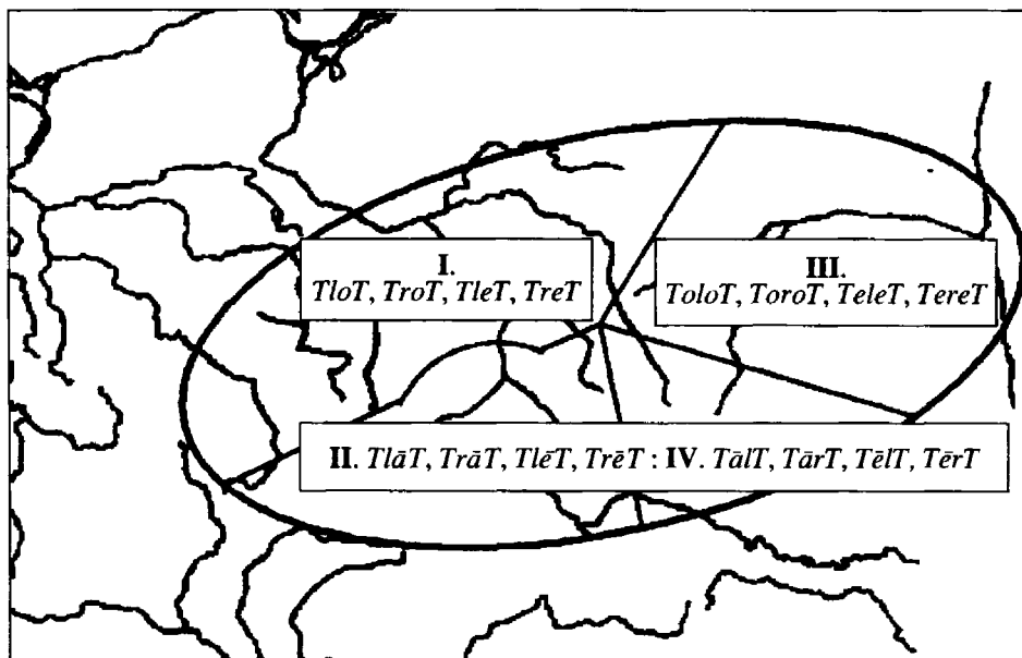
Рис. 2. Метатеза плавных в инлаутных группах: I. Простая метатеза ( TloT, TroT, TleT, TreT ). II. Метатеза с продлением гласных ( TlāT, TrāT, TlēT, TrēT ). III. Ограниченная метатеза/полногласие ( ToloT, ToroT, TeleT, TereT ). IV. Без метатезы, но с продлением гласного, как в II ( TālT, TārT ).
